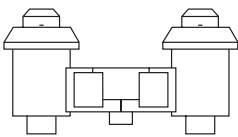
Plano conexión B Conector plano de 6,3 mm protegido ante salpicaduras de agua si se combina con boquilla de goma 9GT 700 452-005
