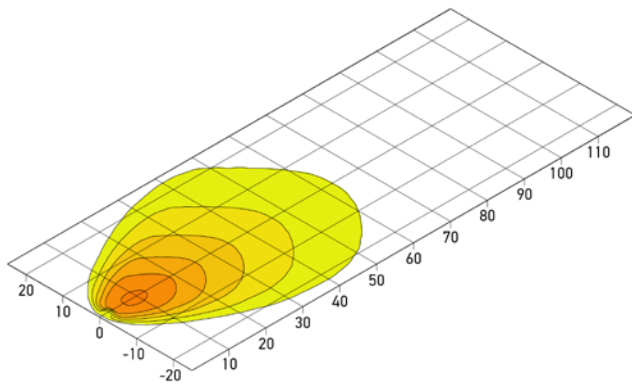
Nahfeldausleuchtung
