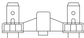
Schema di collegamento A Connettore faston da 6,3 mm
