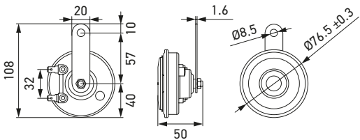
Clacson a disco S90
