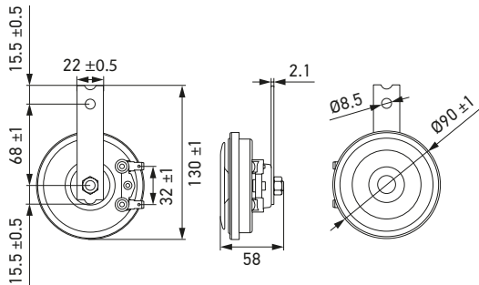
Clacson a disco S92
