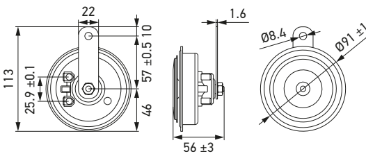
Clacson a disco S92
