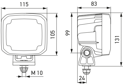
Schéma coté
