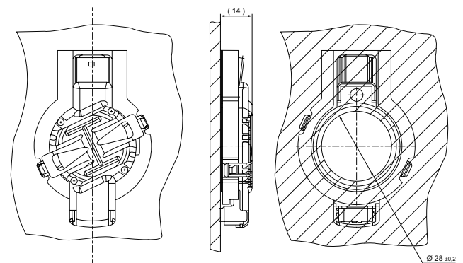
Representación del montaje en el parabrisas
