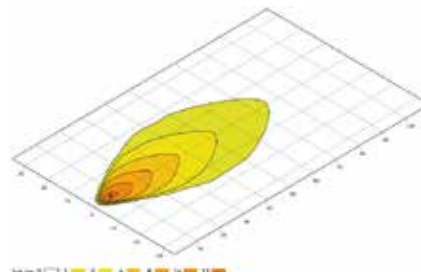
Langtrækkende belysning
