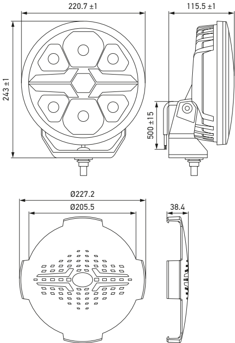
Ostona okrągła, 9 cali (8XS 358 198-011, wyposażenie dodatkowe)
