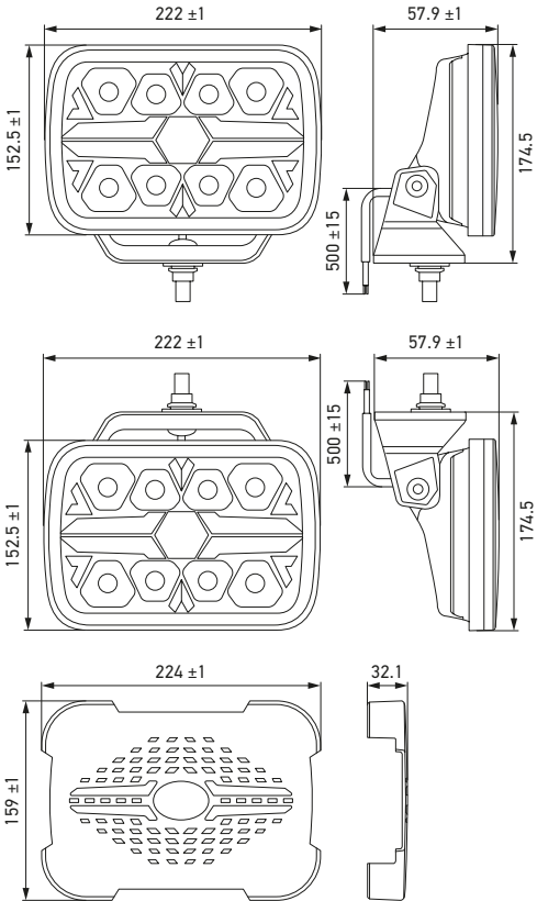
Ostona prostokątna, 9 cali (8XS 358 198-021, wyposażenie dodatkowe)
