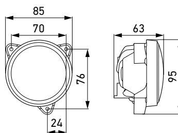
3-Punkt-Einbau
